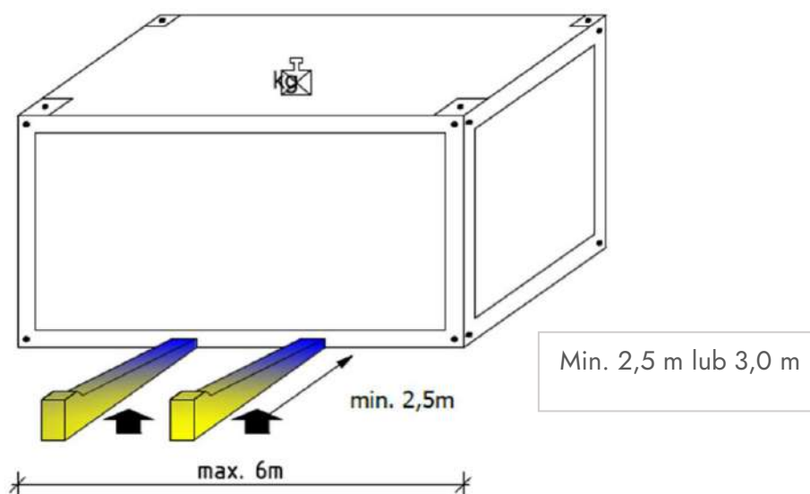
Rys. 5. Minimalna długość widel wózka widłowego – 2,5 m dla kontenerów o szerokości 2,438 m oraz 3,0 m dla kontenerów o szerokości 2,99 m.
