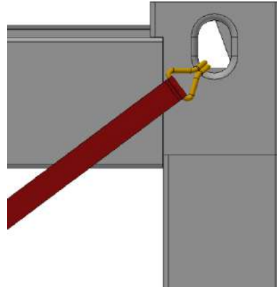
Rys. 2. Sposób zaczepienia pasa transportowego o naroże kontenera.
