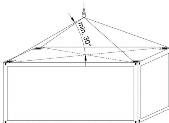
Rys. 3. Minimalny kąt pomiędzy zawiesiem a dachem kontenera.
